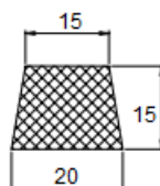
Profil raclete
