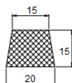
Profil raclete
