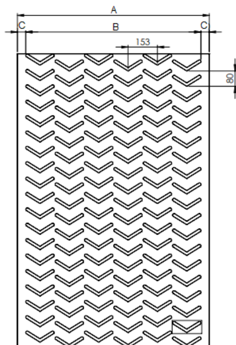
Raclete (dimensiuni)
