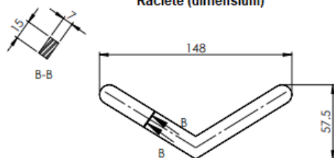
Raclete (dimensiuni)
