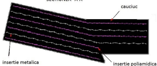
SECTIUNEA "A-A"
