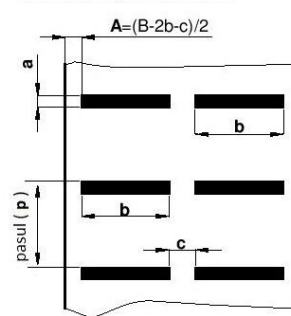
2. Banda transportoare cu racleti transversali pe doua randuri
