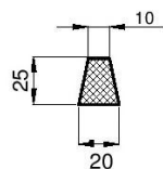
Profil racleti
