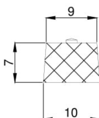
Sectiune raclet V300x7
